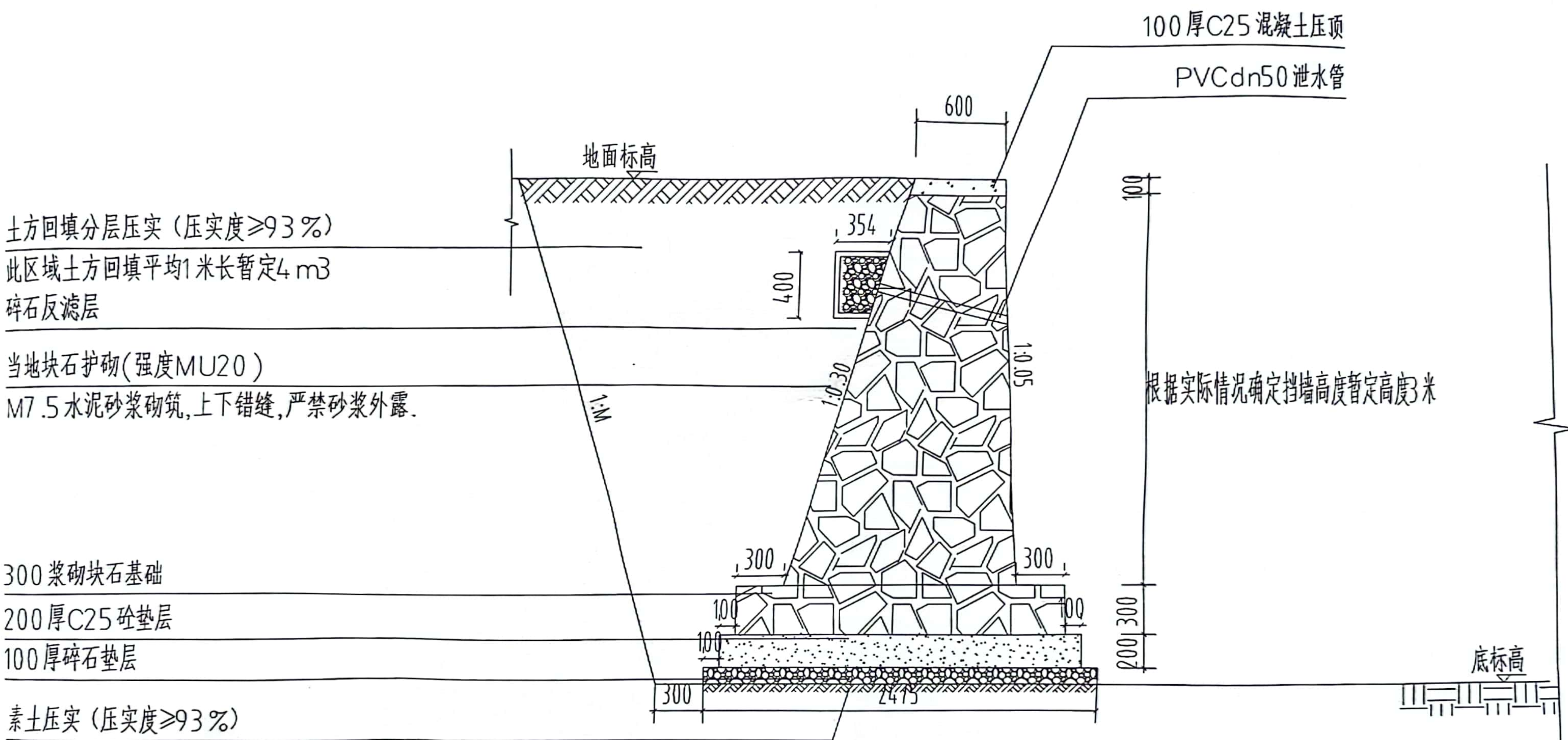
干砌石驳岸详图
